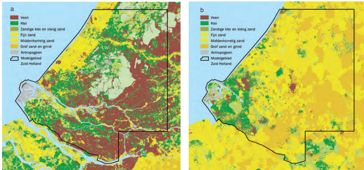
Figuur 3. Lithologische variatie op diepten van 5 m (a) en 20 m (b) onder NAP in Zuid-Holland.
